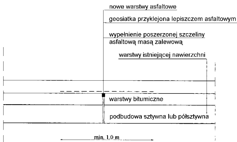
Rys. 5. Naprawa powierzchni pęknięć odbitych z ułożeniem nowych warstw asfaltowych
